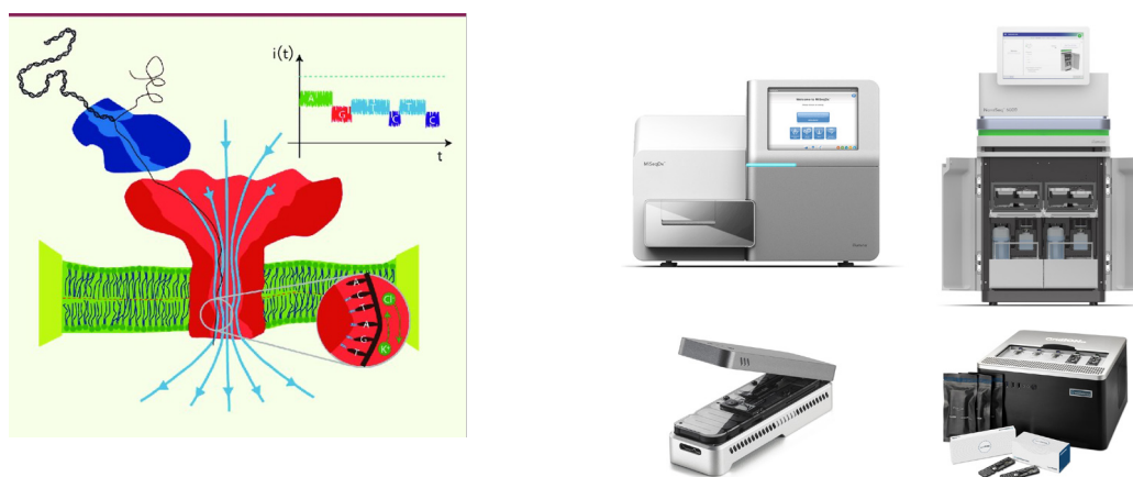
Figure 1.8 Séquençage
